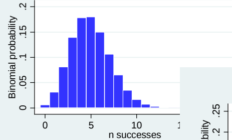
n=100 p=0.05
