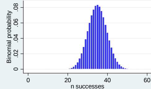
n=100 p=0.35
